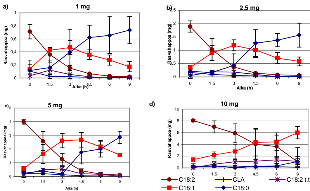
Kuva 2. Linoliyhapon biohydrogenaatioprofiilien keskiarvot ja keskihajonnat eri annostasoilla. a) 1 mg linoliyhappoa, b) 2,5 mg linoliyhappoa, c) 5 mg linoliyhappoa ja d) 10 mg linoliyhappoa. Linoliyhappo (C18:2), konjugoituidu linoliyhapot (CLA), ei-konjugoituidu C18:2 –isomeerit (C18:2 t,t), C18:1 monoeneit (C18:1) ja steariiniyhappo (C18:0).
