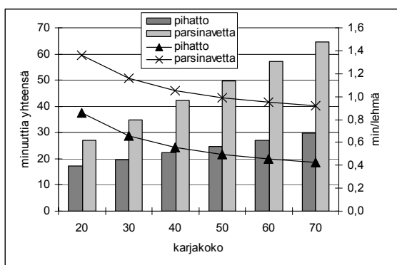
Kuvio 1. Karjakoon vaikutus eläinten siirtoon kuluvaan aikaan (ei henkilötyöaika) parsinavetassa ja pihatossa, laitumen etäisyys 200 metriä. Ajat sisältävät yhteen lypsykertaan liittyvien eläinten siirtojen työajat.
