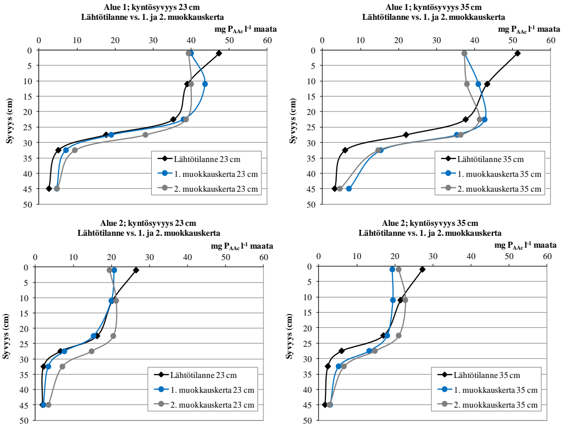
Kuva 2. Maan helppoliukaisen fosforin keskimääräiset pitoisuudet (viljavuus-P; P AAc , mg l -1 maata) eri syvyyksissä. Pitoisuudet on määritetty näytteenottoalueiden 1 ja 2 lähtötilannetta kuvaavista maanäytteistä sekä seuranta-äytteistä, jotka on otettu syksyllä 2011 (1. muokkauskerta) ja syksyllä 2012 (2. muokkauskerta) noin 23 cm:n ja noin 35 cm:n syvyyteen kynnetyltä lohkolta. Alue 1 = korkean fosforiluokan maa, alue 2 = hyvän fosforiluokan maa. (Alueelta 1 kerranne 4 on poistettu analyysistä.)
